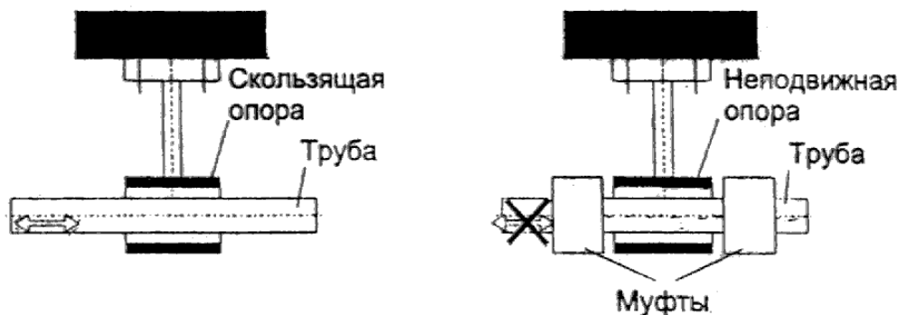
Рис. 4.1. Виды опор
