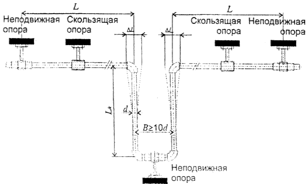
Рис. 2.5. П-образный компенсатор
