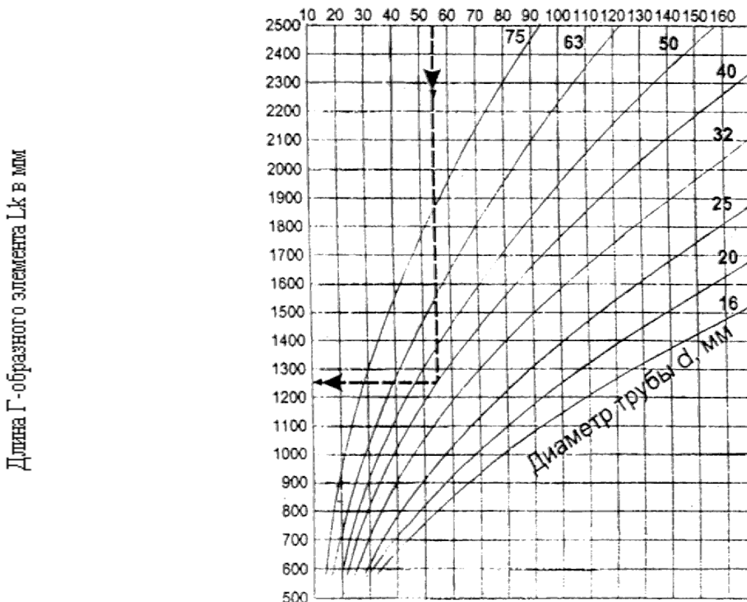
Рис. 2.7. Номограмма для определения длины участка трубы, воспринимающего тепловое удлинение
