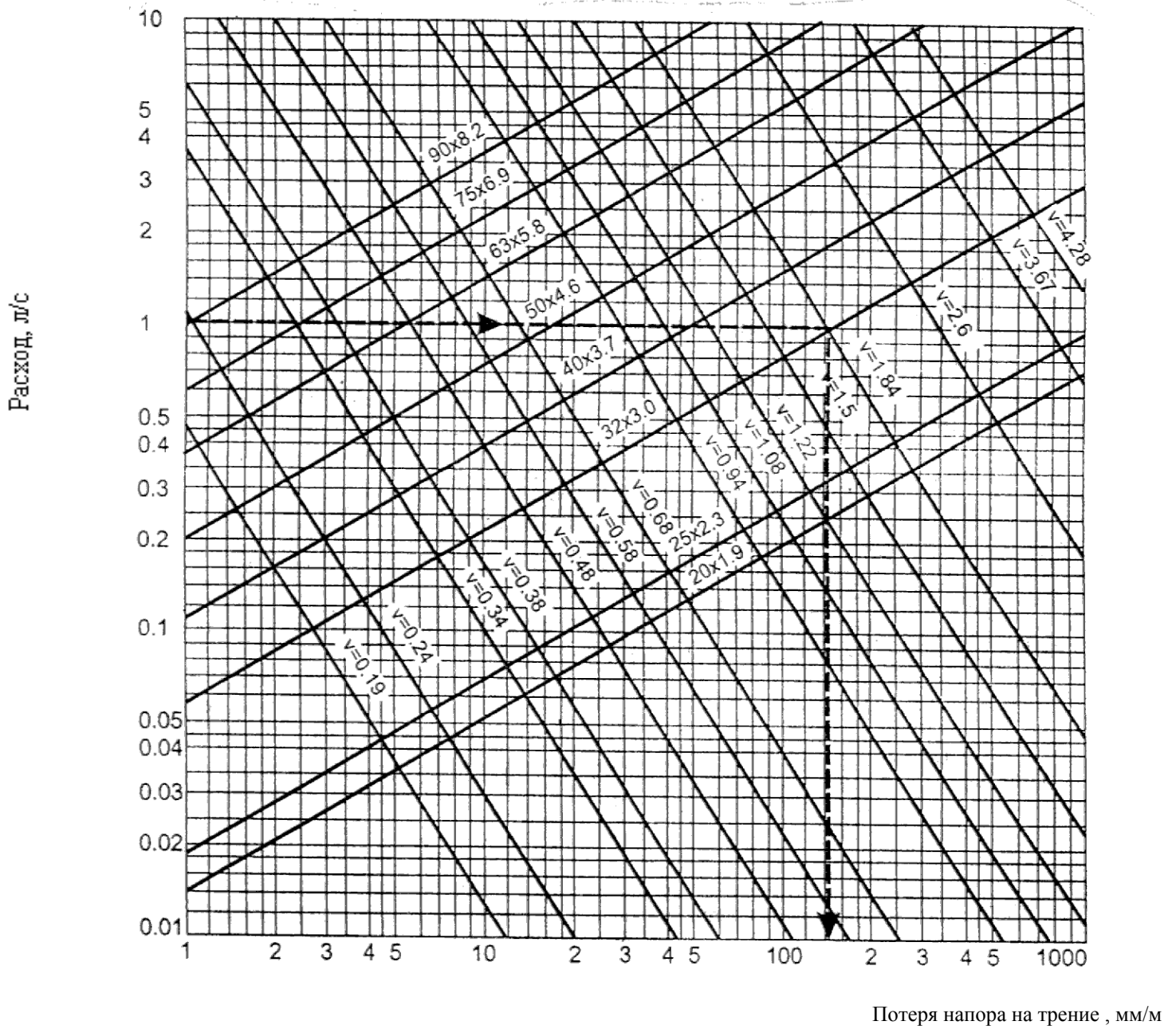
Рис. 2.1. Номограмма для инженерного гидравлического расчета холодного водопровода из труб PPRC (PN10)
