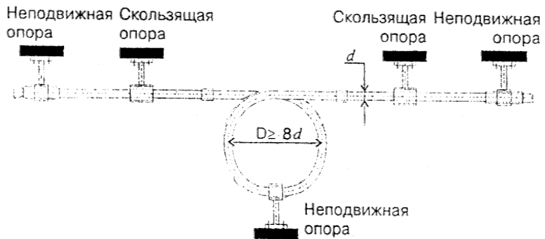
Рис. 2.6. Петлеобразный компенсатор
